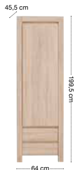
skříňka REG1D2SL
