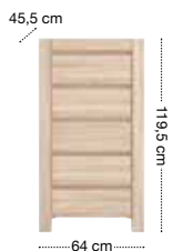
komoda KOM5S
