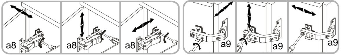
Regulacja drzwi / Seřizování frontálních dílů / Adjustment of door Az előrészek szabályozása / Nastavenie číel
